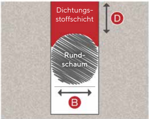
B= Fugenbreite D= Fugentiefe
